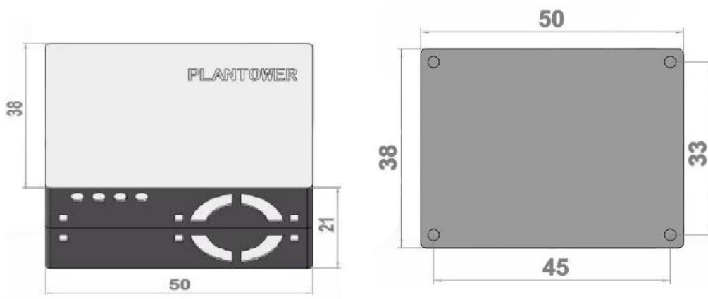
图 3 外形尺寸图
